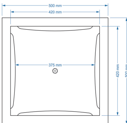
Botanic 50 Innenansicht inkl. Bemaßung
