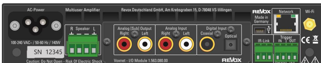
Abb.: M30 mit installiertem I/O Modul
