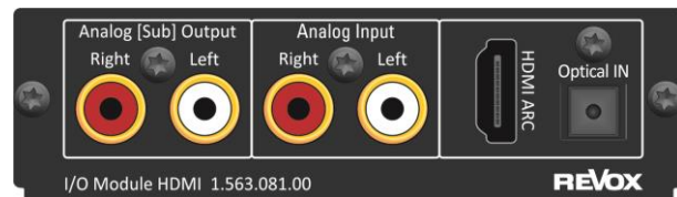
Abb.: I/O-HDMI Modul
