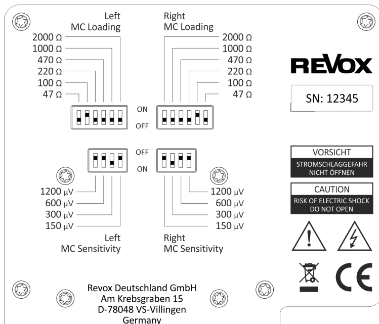
Abb: Werkseinstellung Phono­vorverstärker für Ortofon Quintet Bronze/ Black
