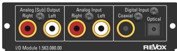
Fig.: I/O module
